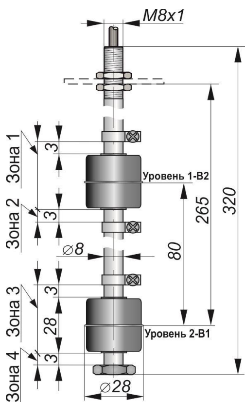
Габаритный чертеж
