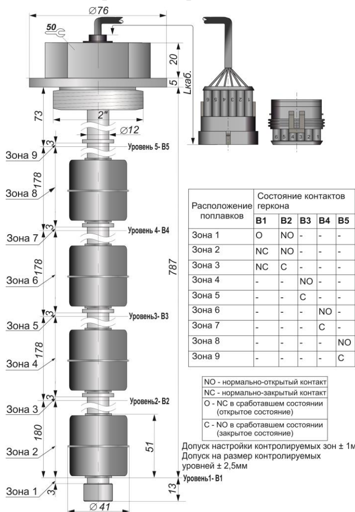
Габаритный чертеж
