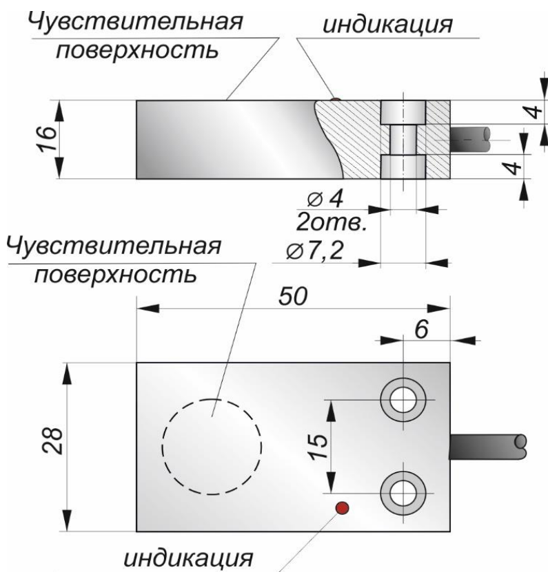
Габаритный чертеж
