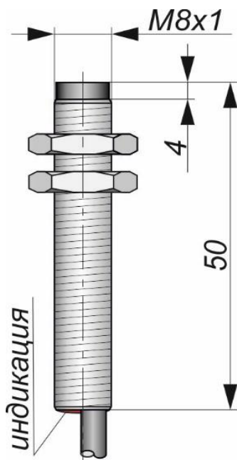
Габаритный чертеж
