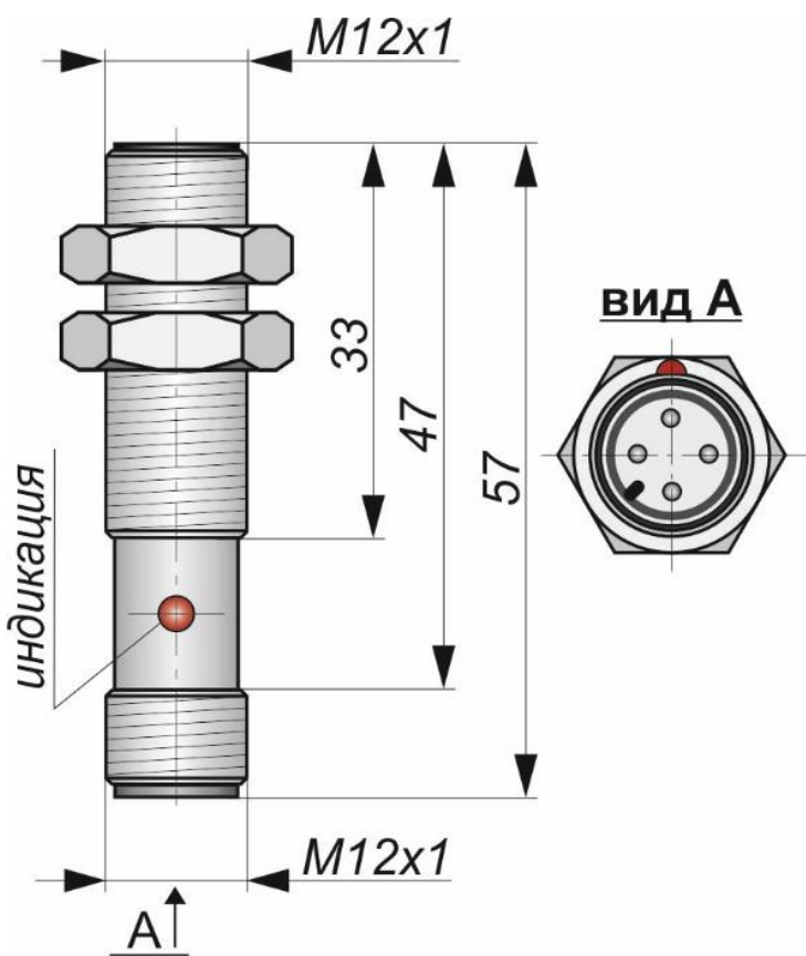
Габаритный чертеж
