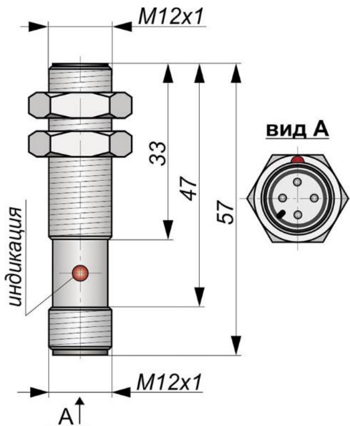
Габаритный чертеж
