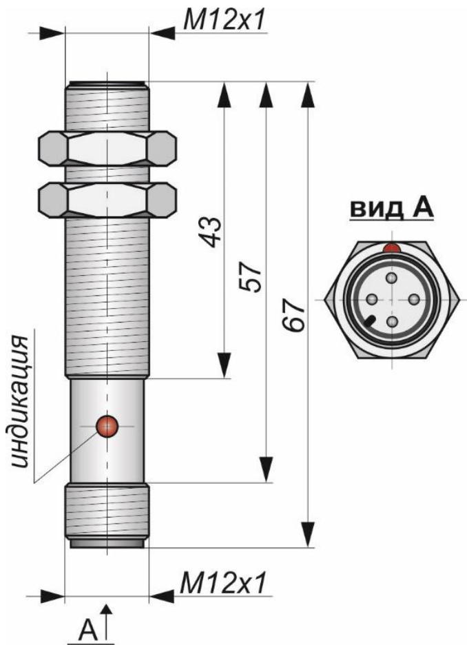
Габаритный чертеж
