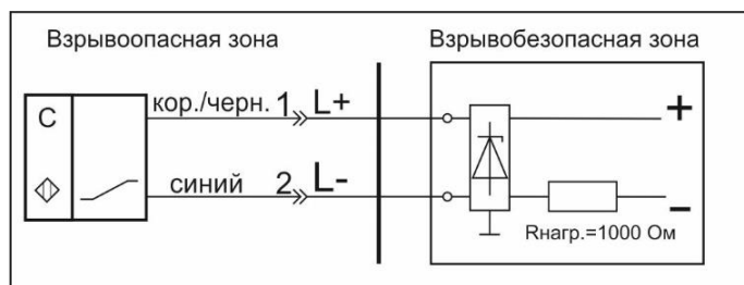
Схема соединения
