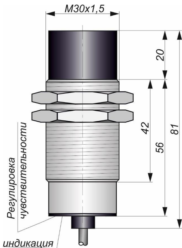
Габаритный чертеж
