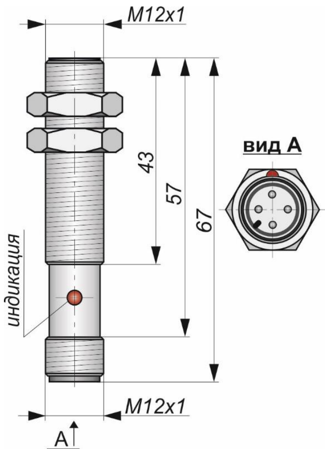
Габаритный чертеж
