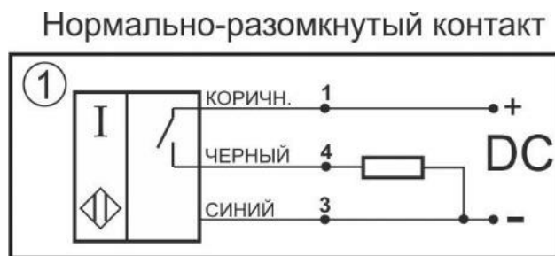
Схема соединения
