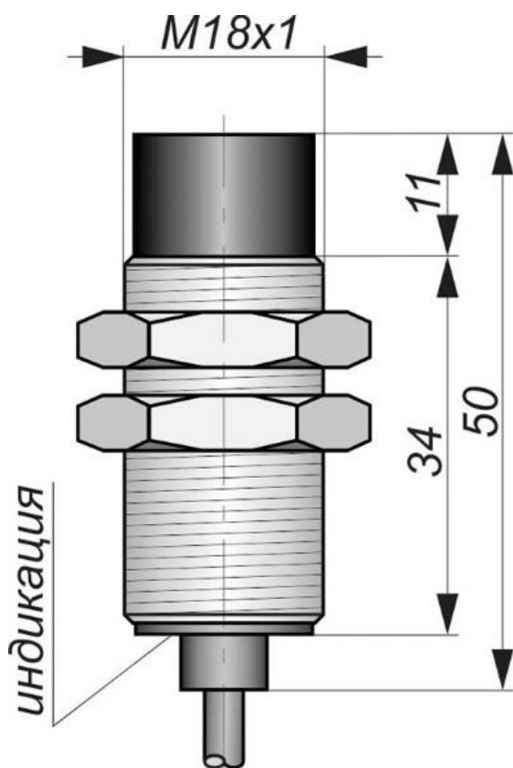
Габаритный чертеж
