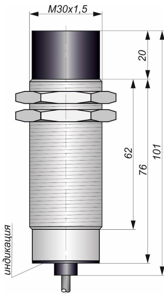
Габаритный чертеж
