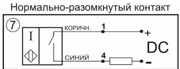
Схема соединения
