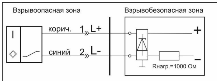
Схема соединения
