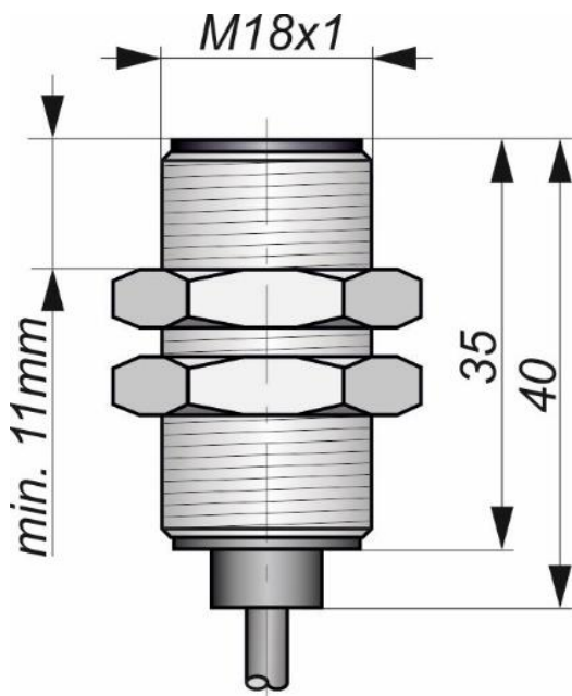
Габаритный чертеж
