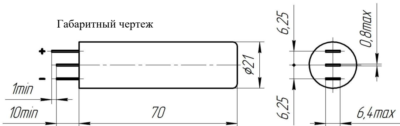
Нормально-разомкнутый контакт
